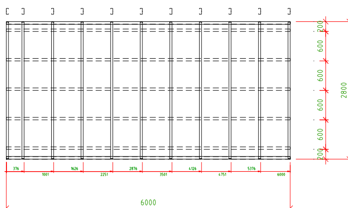
ADTtools – montážní schéma
