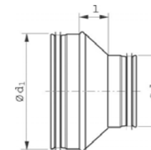
RCU-d1-d2 centrikus szűkítő, Safe
