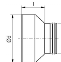
RCFU-d-d2 centrikus szűkítő, female csatlakozással, Safe
